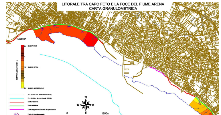
SEDIMENTOLOGICAL SURVEY
