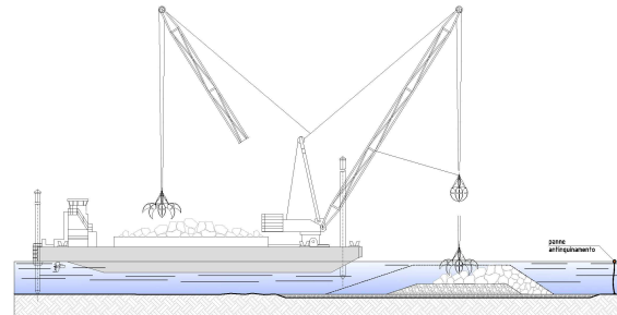
SEZIONE E-E - Posa massi di III categoria
